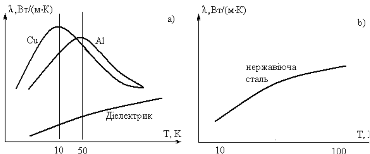
Рис. 1.2 Залежність коефіцієнту теплопровідності від температури: а) чисті матеріали та діелектрики, б) сплави.
