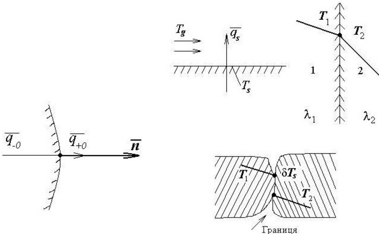
Рис. 1.5 До визначення граничних умов 3-го роду
