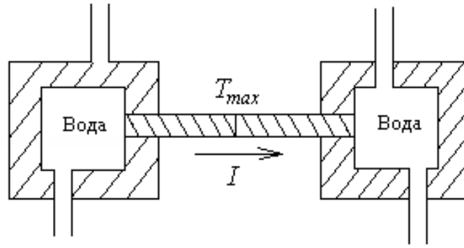
Рис. 3.6 Метод Кольрауша
